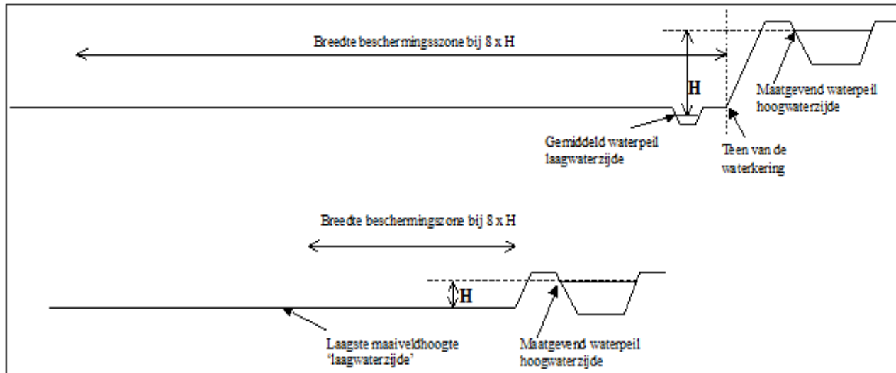
Figuur: Waterkerende hoogte
