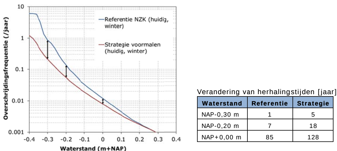
Figuur 4: Illustratie van de manier waarop de verandering in faalkans voor de Slim Watermanagement strategieën in beeld is gebracht. De berekende overschrijdingsfrequenties zijn voor drie kenmerkende waterstanden uitgelezen, omgezet naar herhalingsstijden en vergeleken met de referentiesituatie.
