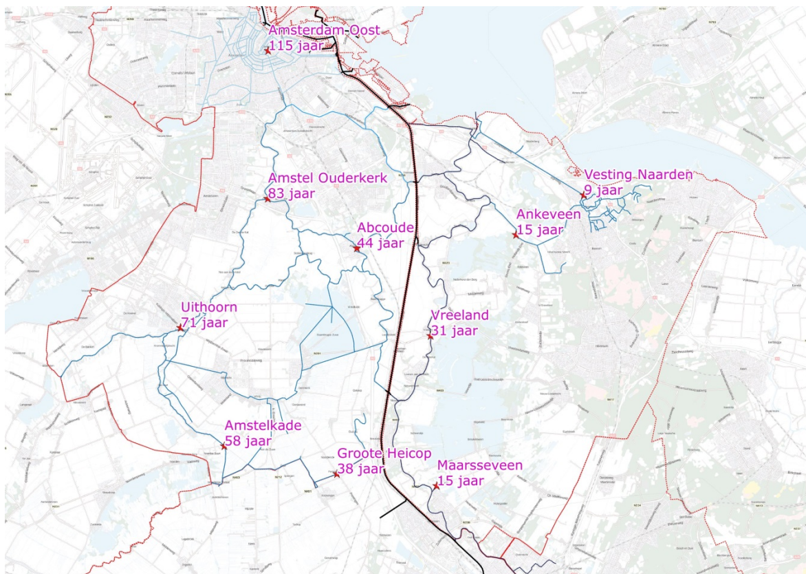
Figuur 7: De berekende gemiddelde herhalingstijden van een waterstand van NAP+0,00 m op tien locaties in het watersysteem (locaties Ankeveen en Vesting Naarden liggen op de s'Gravelandsevaart-boezem en hebben een hoger toetspeil).
