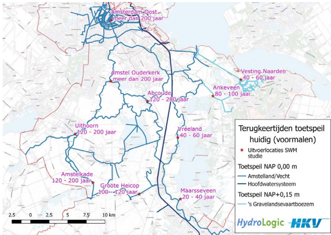
Figuur 2: Terugkeertijden van toetspeil op de boezem van AGV met voormalen (maatregel Slim Watermanagement).
