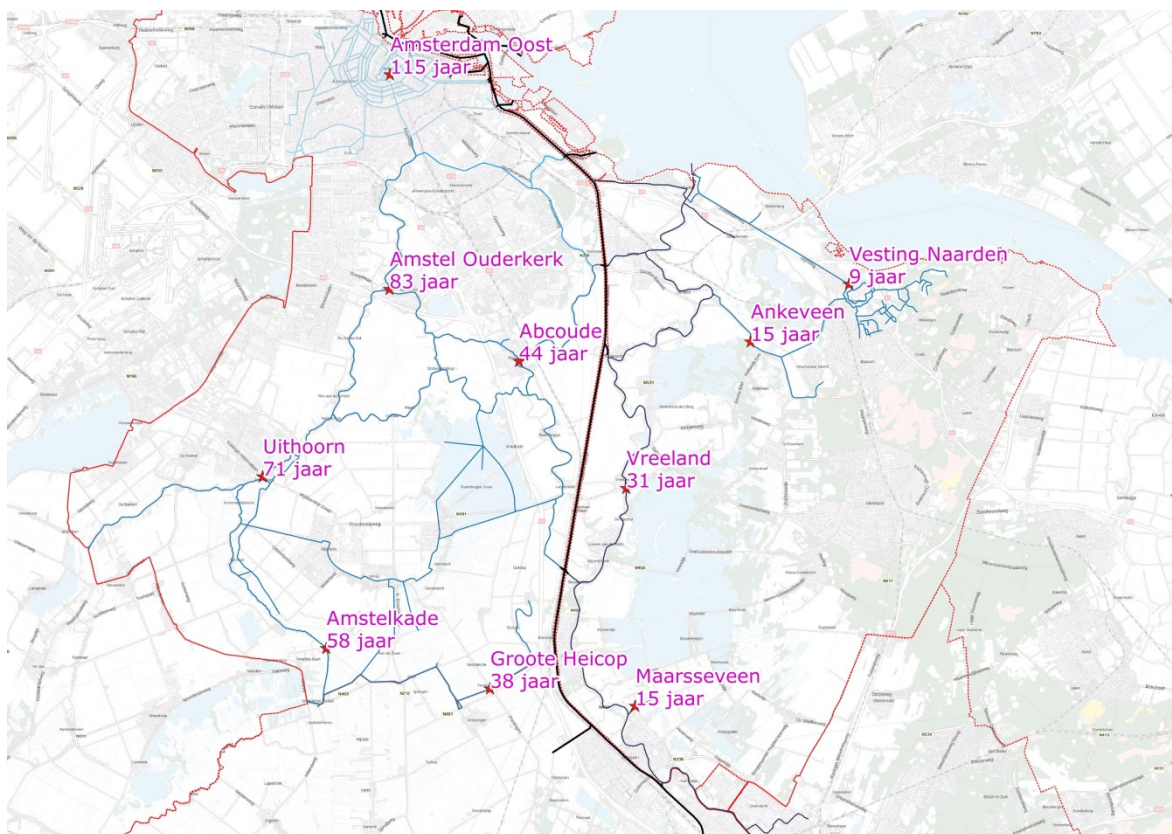
Figuur 2: De berekende gemiddelde herhalings tijden van een waterstand van NAP+0,00 m op tien locaties in het watersysteem (locaties Ankeveen en Vesting Naarden liggen op de 's Gravelandsevaart-boezem en hebben een hoger toetspeil).
