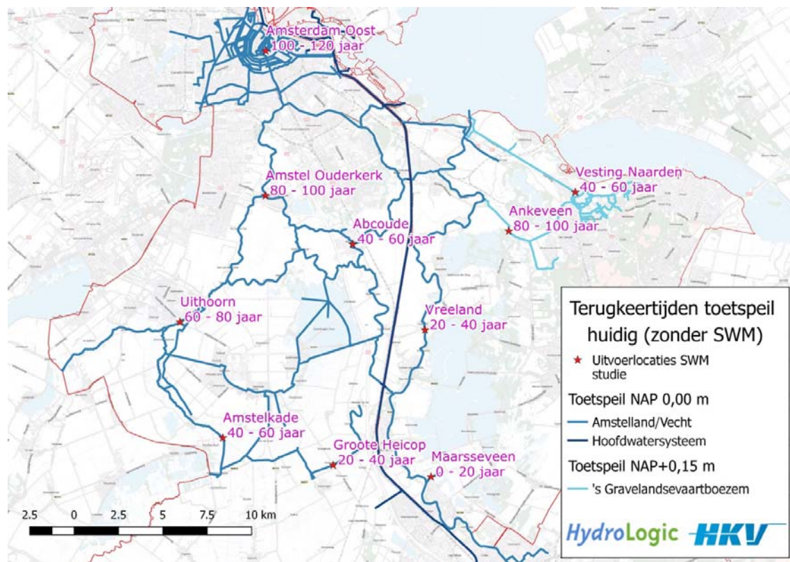
Figuur 1: Terugkeertijden van toetspeil op de boezem van AGV zonder toepassen Slim Watermanagement.
