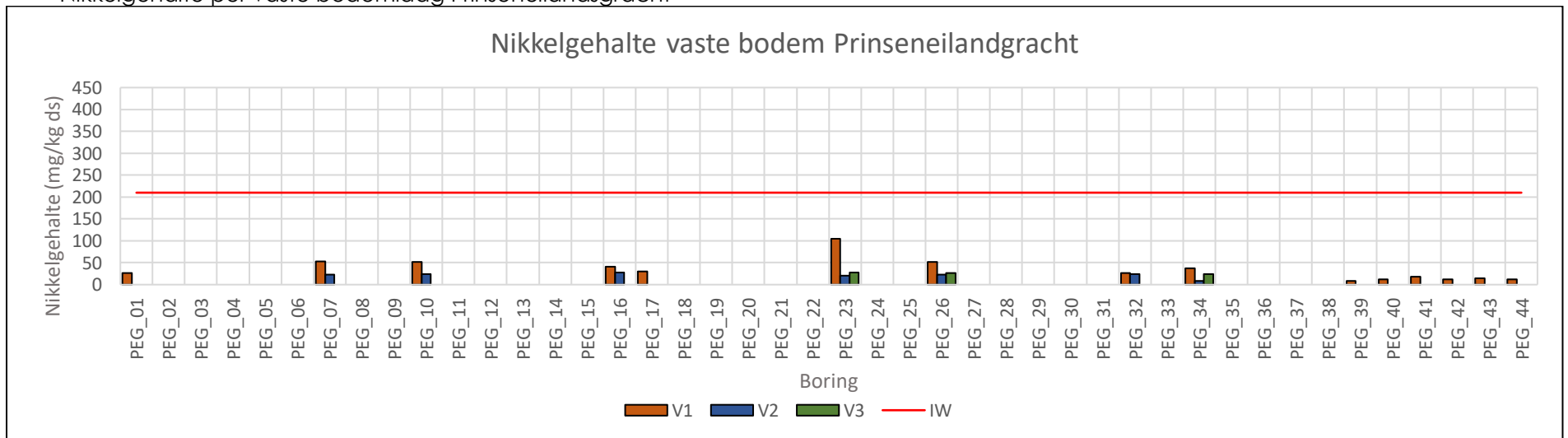
Nikkelgehalte per vaste bodemlaag Prinseneilandsgracht
