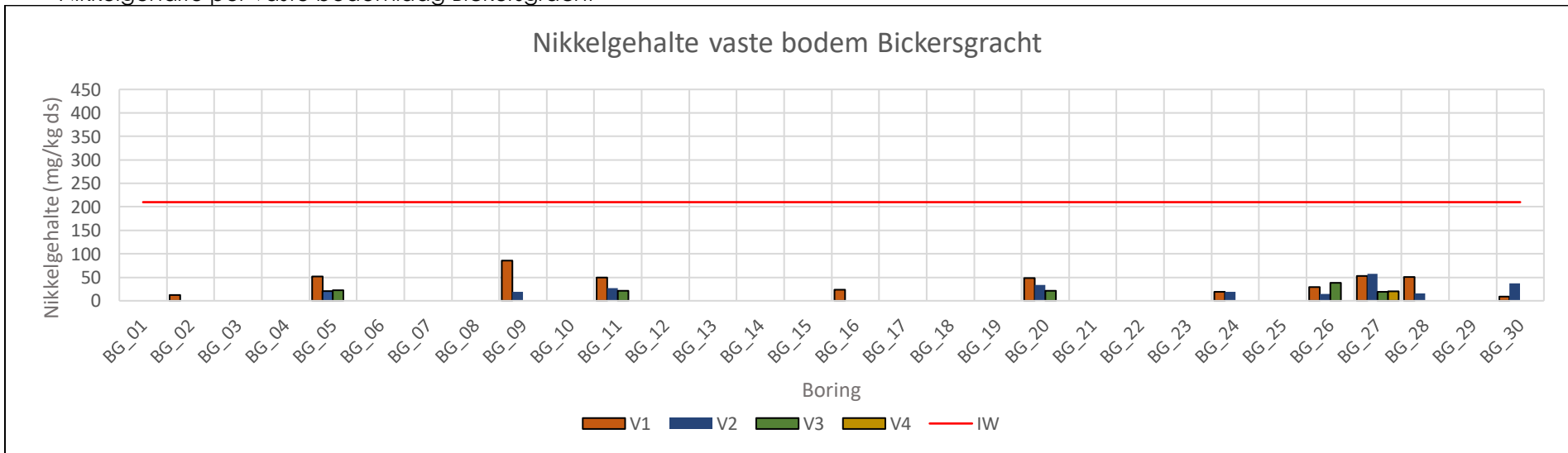
Nikkelgehalte per vaste bodemlaag Bickersgracht
