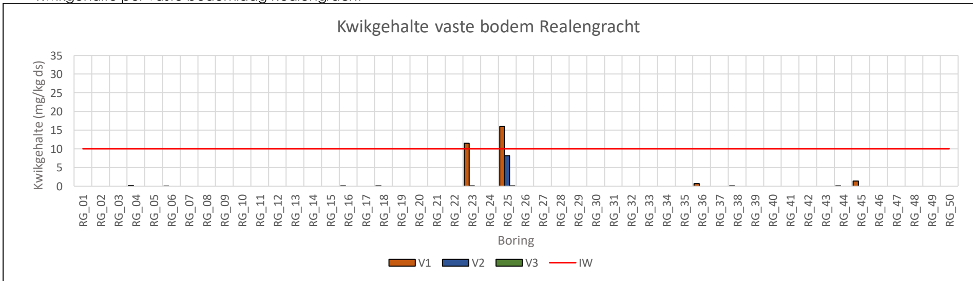
Kwikgehalte per vaste bodemlaag Realengracht
