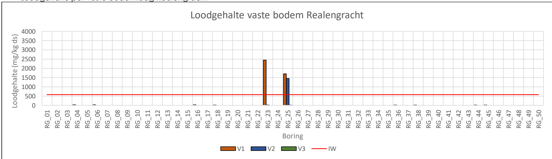
Loodgehalte per vaste bodemlaag Realengracht
