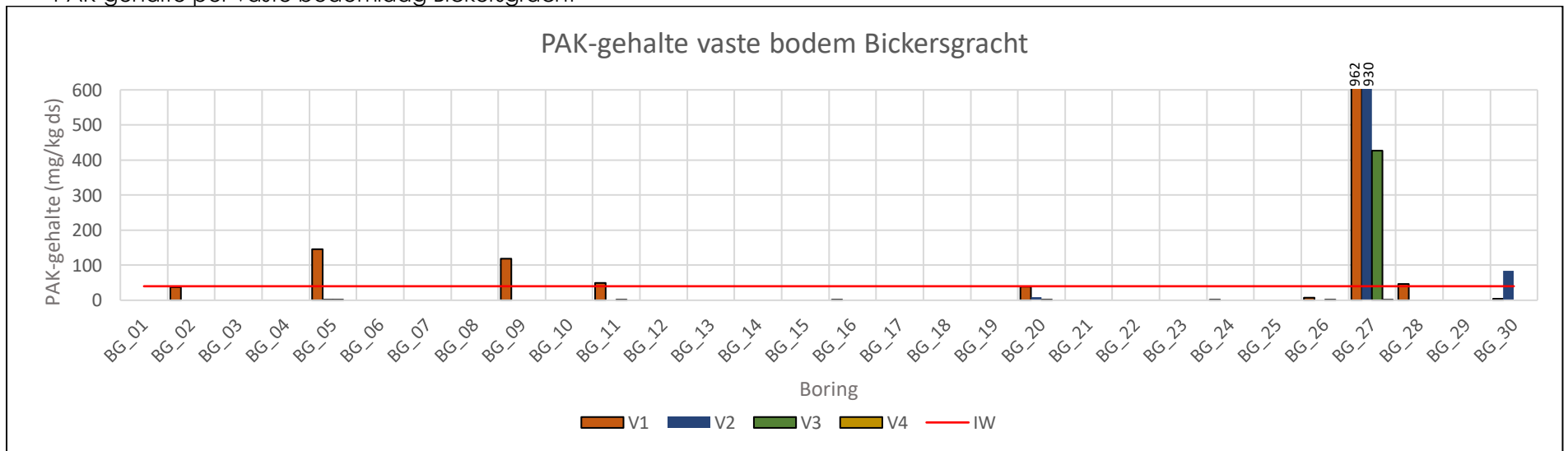
PAK-gehalten per vaste bodemlaag Bickersgracht
