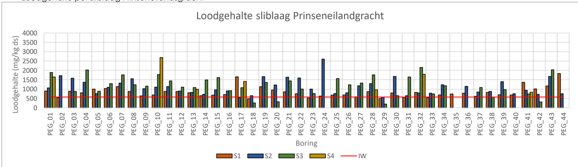
Loodgehalte per sliblaag Prinseneilandsgracht
