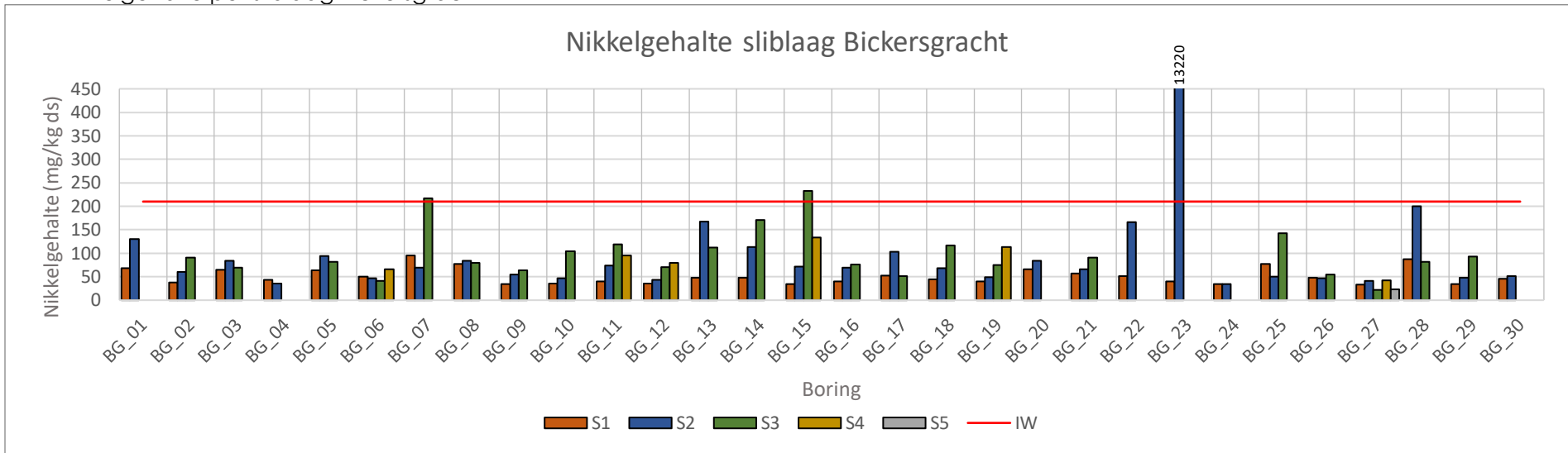
Nikkelgehalte per sliblaag Bickersgracht
