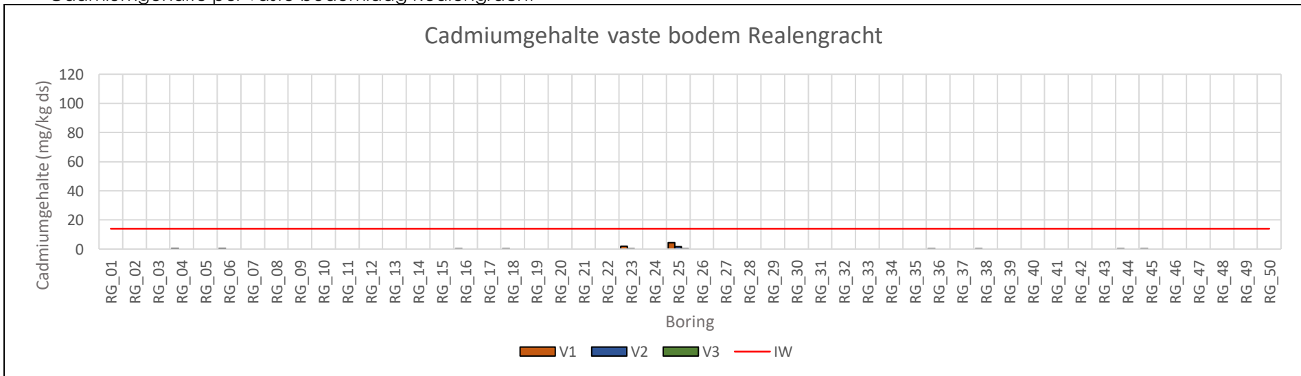
Cadmiumgehalten per vaste bodemlaag Realengracht
