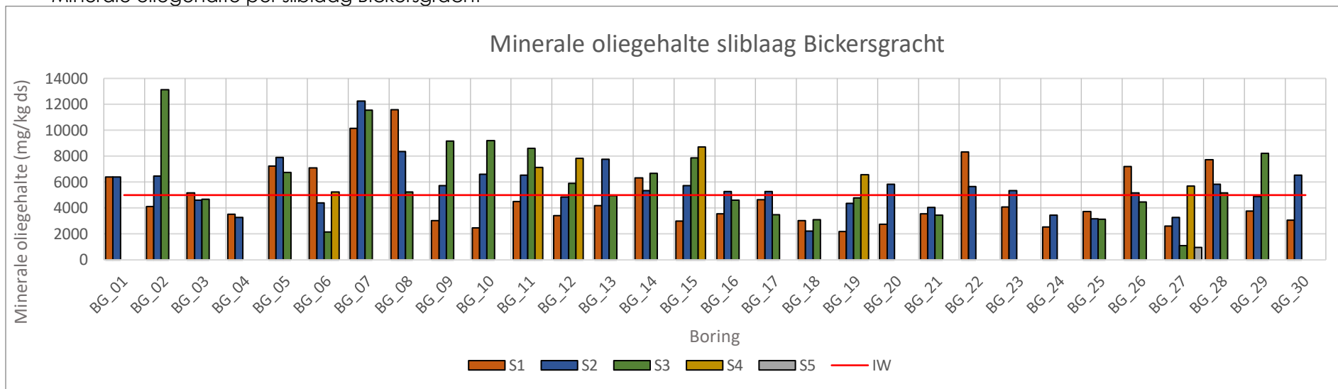
Minerale oliegehalte per sliblaag Bickersgracht
