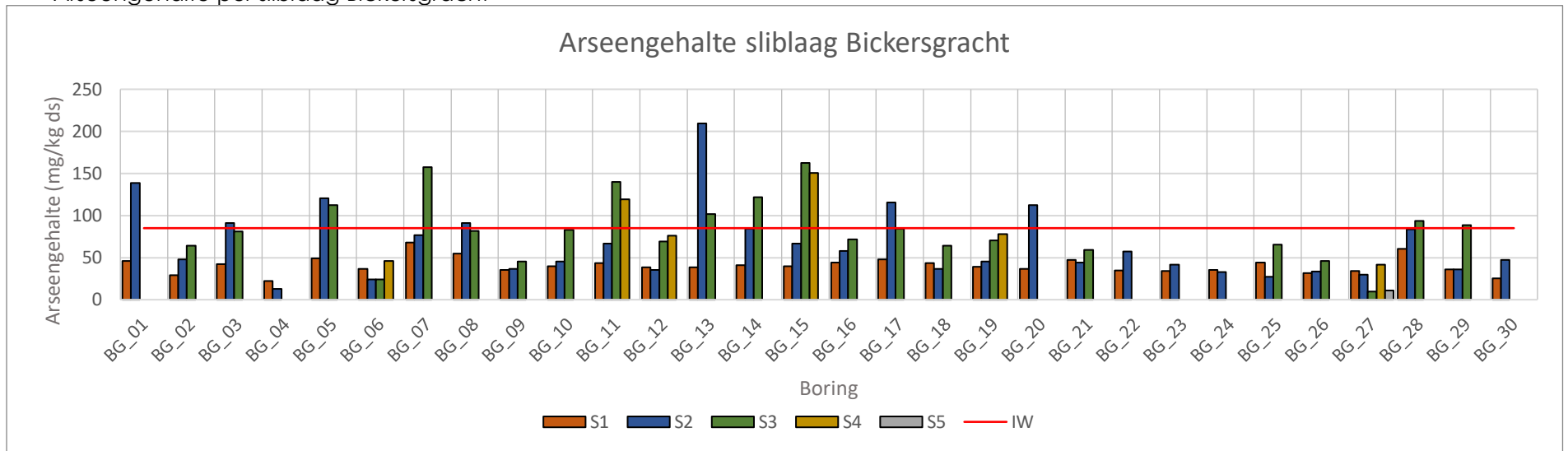
Arseengehalte per sliblaag Bickersgracht
