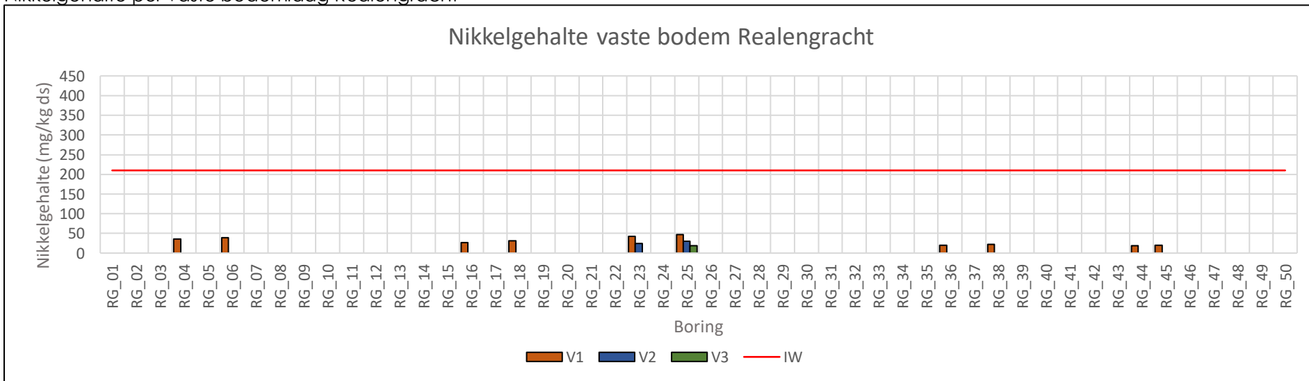
Nikkelgehalte per vaste bodemlaag Realengracht
