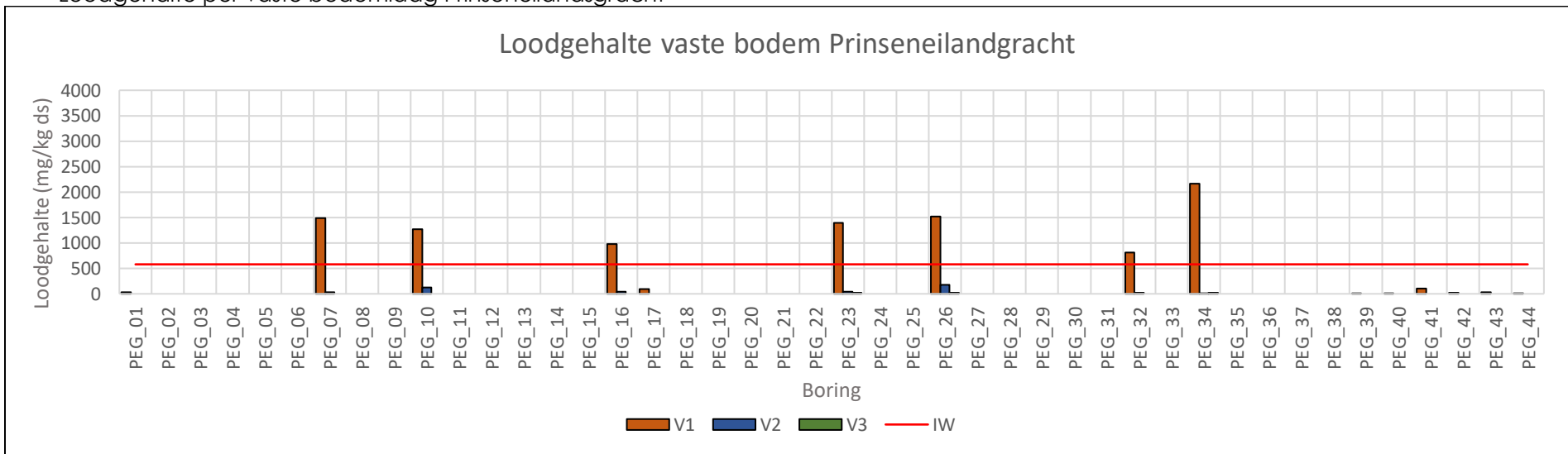
Loodgehalte per vaste bodemlaag Prinseneilandsgracht
