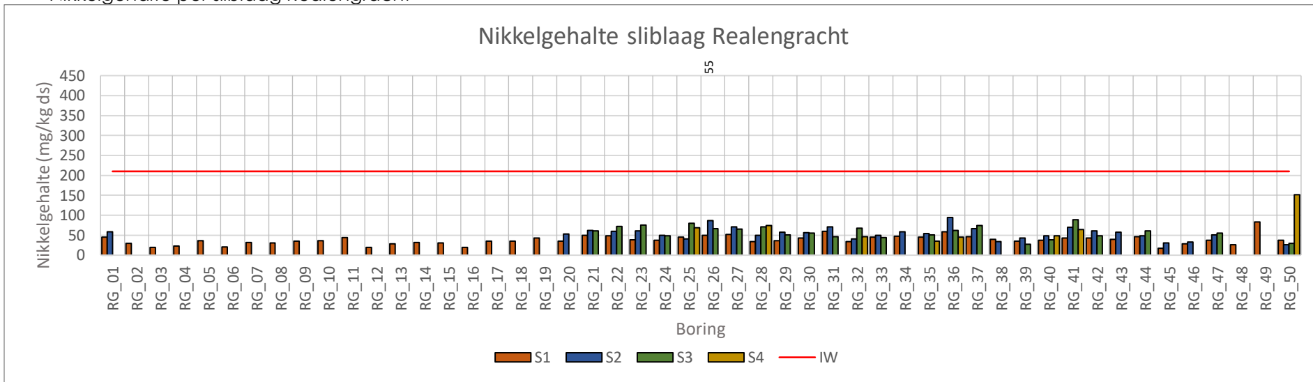
Nikkelgehalte per sliblaag Realengracht
