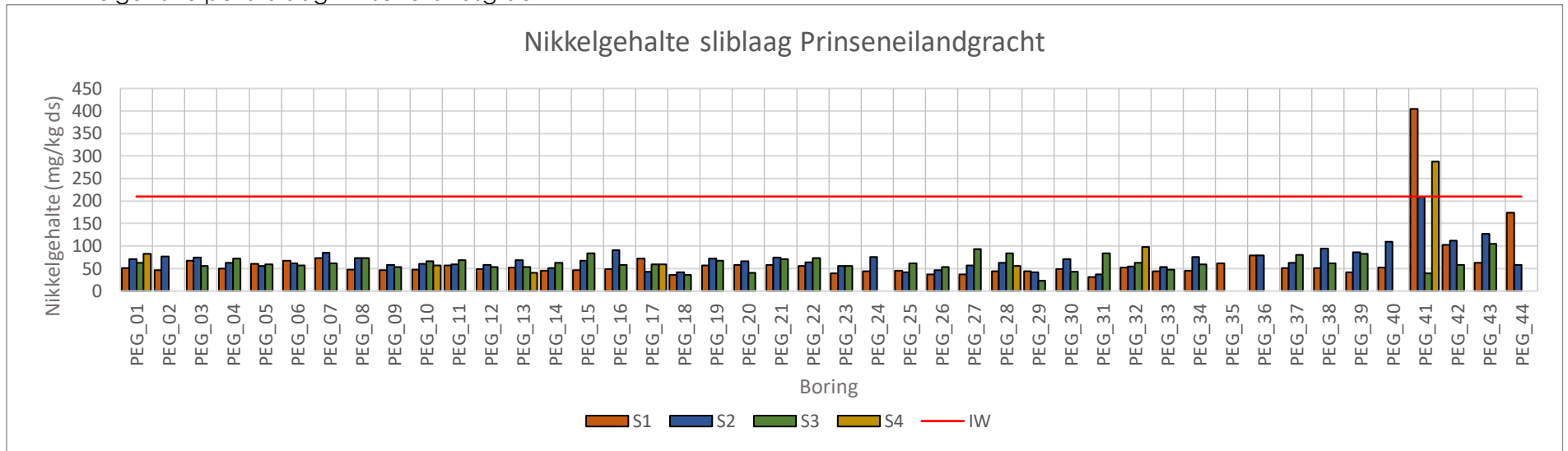
Nikkelgehalte per sliblaag Prinseneilandsgracht
